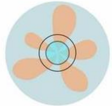
Kvantmekanisk modell
