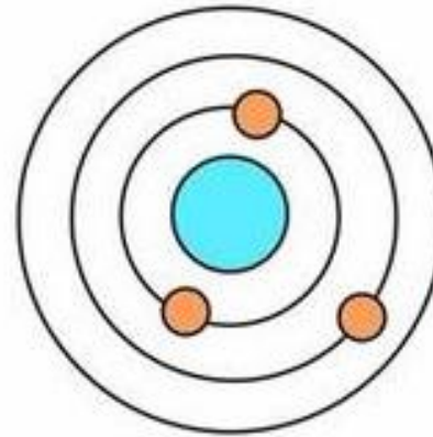
Bohr
